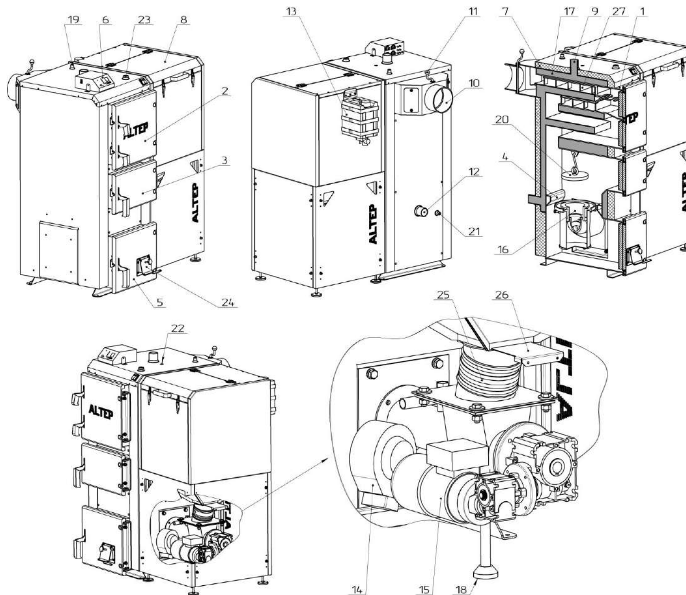
Рисунок 2 – Внешний вид и основные элементы котла
