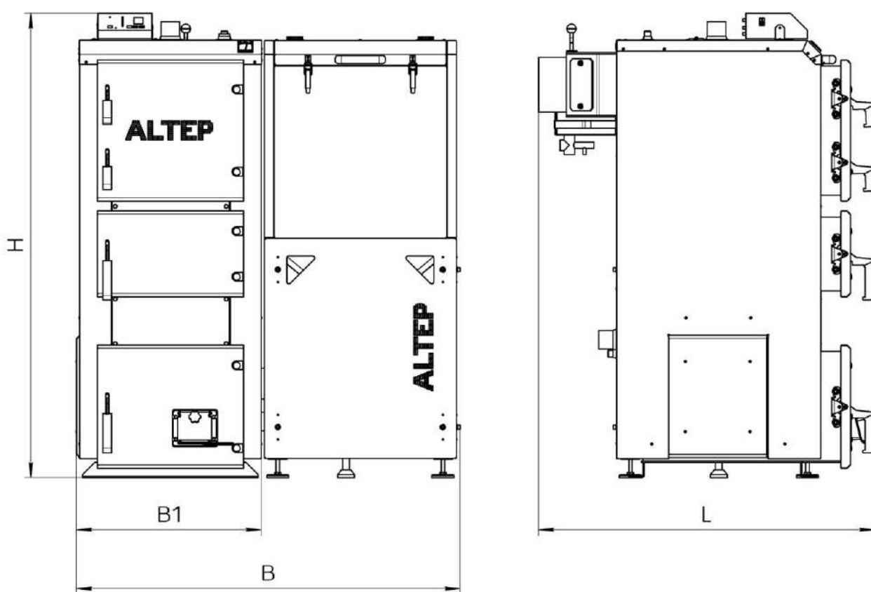
Рисунок 1 – Габаритный чертеж котла типа КТ-2Е-SH
