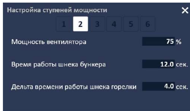
Двухшнековый способ
