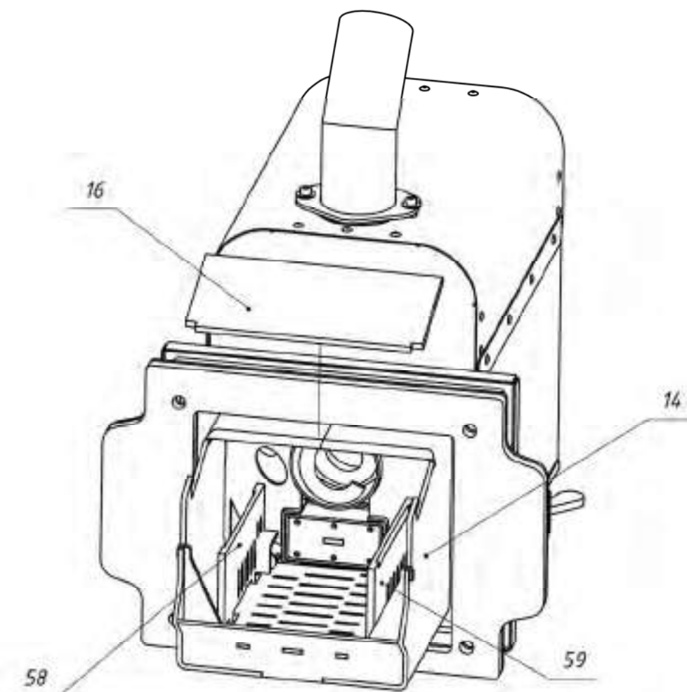
Рис. 75 Поворачивая боковины колосника (поз. 58 и 59), в сторону центра камеры сгорания установить их вертикально.
