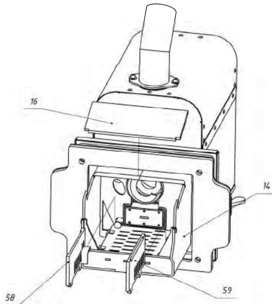
Рис. 70 Вынуть из камеры сгорания дощевину колосника (поз. 58 и 59).
