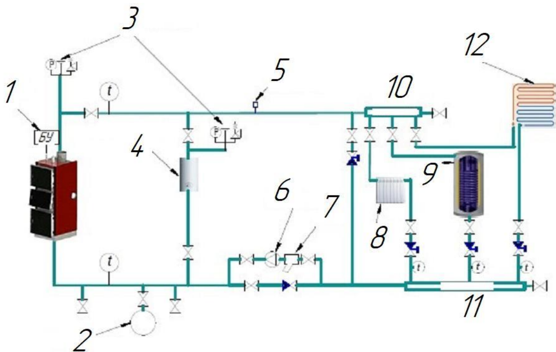
Рисунок 5 – Типовая схема обвязки котла. 1-блок управления котлом; 2-расширительный бак; 3-группа безопасности; 4-электродкотел резервный; 5-воздухоотводчик; 6-насос циркуляционный; 7-фильтр; 8-радиатор; 9-бойлер; 10-коллектор подачи; 11-коллектор обратной подачи; 12-теплый пол
