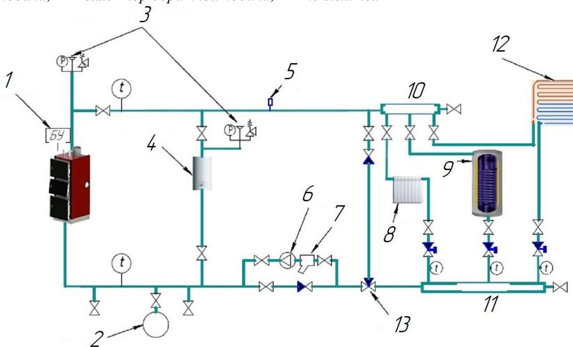
Рисунок 5 – Типовая схема обвязки котла. 1-блок управления котлом; 2-расширительный бак; 3-группа безопасности; 4-электродкотел резервный; 5-воздухоотводчик; 6-насос циркуляционный; 7-фильтр; 8-радиатор; 9-бойлер; 10-коллектор подачи; 11-коллектор обратной подачи; 12-теплый пол
