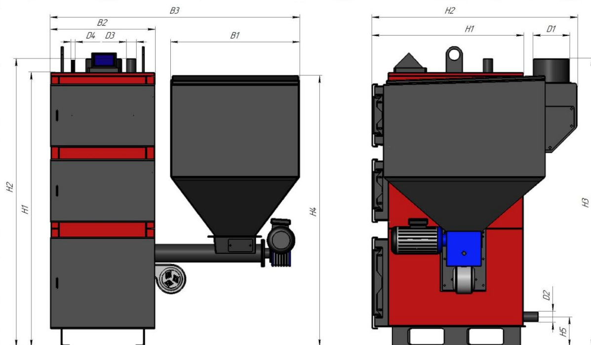
Схема для таблицы размеров VULKAN Eko, Eko Plus
