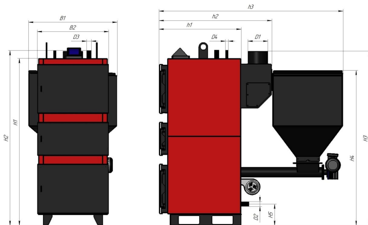
Схема для таблицы размеров VULKAN EKO-Z
