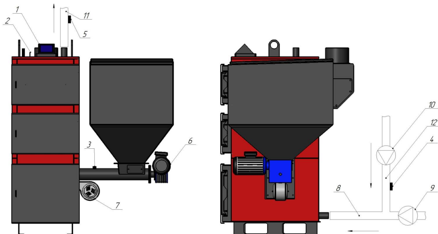
Рисунок 11 — Схема подключения блока управления к котлу. 1-контроллер (подключается к сети 220В); 2-датчик системы отопления (устанавливается в гильзу); 3-датчик шнека; 4-датчик горячего водоснабжения (ГВС); 5-аварийный датчик (термик); 6-мотор-редуктор; 7-вентилятор наддува; 8-труба обратной линии от отопления; 9-насос системы отопления; 10-насос ГВС; 11-труба подачи; 12-труба обратной линии от бойлера ГВС.
