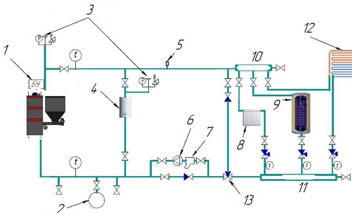
Рисунок 9 — Схема обвязки автоматического котла с трехходовым клапаном. 1-блок управления котлом; 2-расширительный бак; 3-группа безопасности; 4-электродогреватель резервный; 5-воздухоотводчик; 6-насос циркуляционный; 7-фильтр; 8-радиатор; 9-бойлер; 10-коллектор подачи; 11-коллектор обратной подачи; 12-теплый пол; 13-клапан трехходовой.
