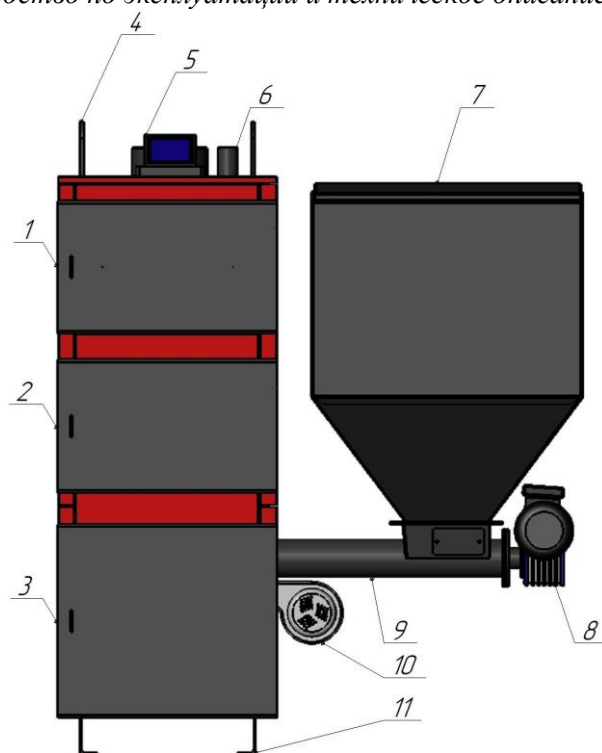
Рисунок 4 — Схема размещения составных элементов в котлах серии Еко, Еко PLUS (Вид спереди). 1-дверь верхняя; 2-дверь средняя; 3-дверь нижняя; 4-ухо транспортировочное; 5-контроллер; 6-труба подачи; 7-бункер; 8-мотор-редуктор; 9-труба топливоподачи; 10-вентилятор наддува; 11-опора котла.
