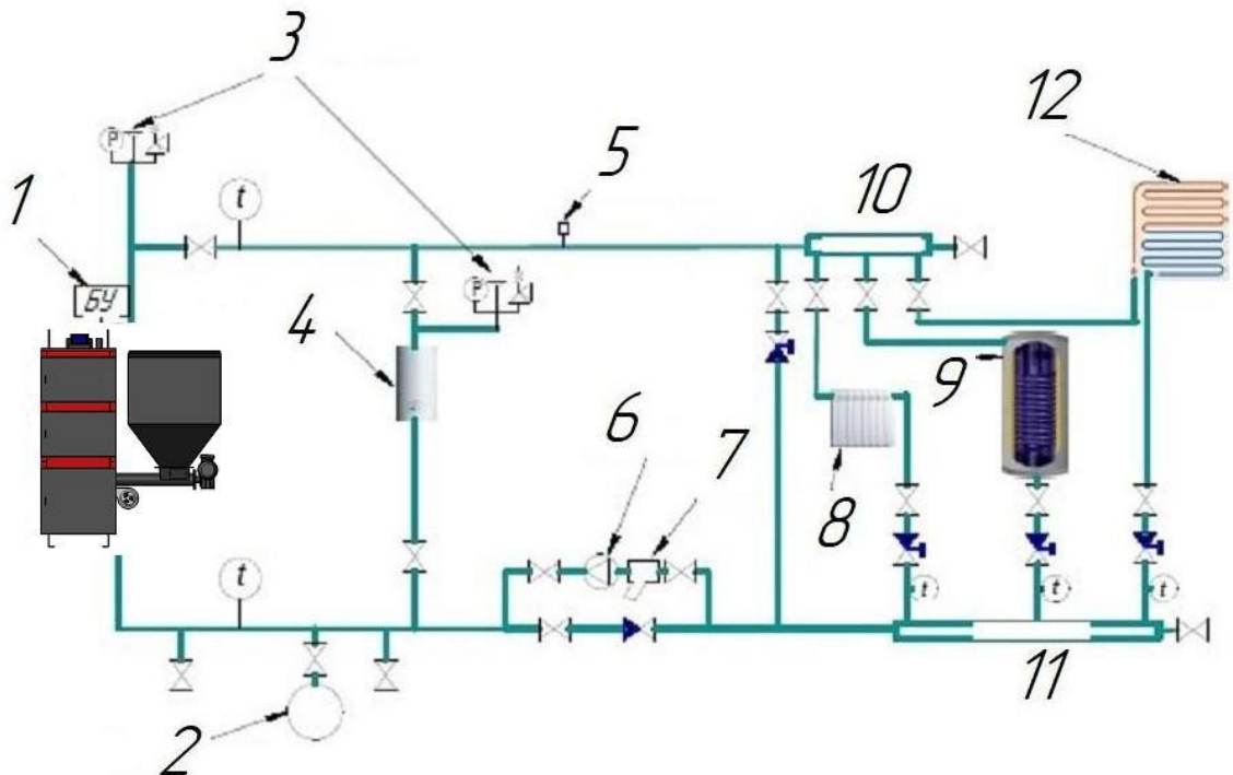
Рисунок 8 — Типовая схема обвязки автоматического котла. 1-блок управления котлом; 2-расширительный бак; 3-группа безопасности; 4-электрокотел резервный; 5-воздухоотводчик; 6-насос циркуляционный; 7-фильтр; 8-радиатор; 9-бойлер; 10-коллектор подачи; 11-коллектор обратной подачи; 12-теплый пол
