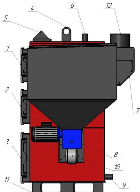
Рисунок 5 — Схема размещения составных элементов в котлах серии Еко, Еко PLUS (Вид сбоку). 1-дверь верхняя; 2-дверь средняя; 3-дверь нижняя; 4-ухо транспортировочное; 5-контроллер; 6-труба подачи; 7-короб дымохода; 8-мотор-редуктор; 9-труба обратной линии; 10-вентилятор наддува; 11-опора котла; 12-дымовая труба.
