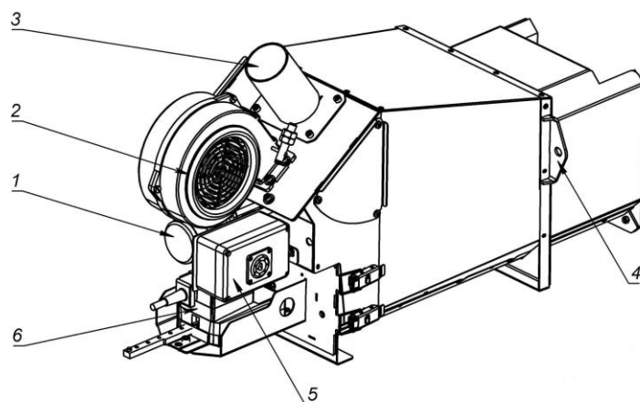
Рис. 4 – Устройство горелки
