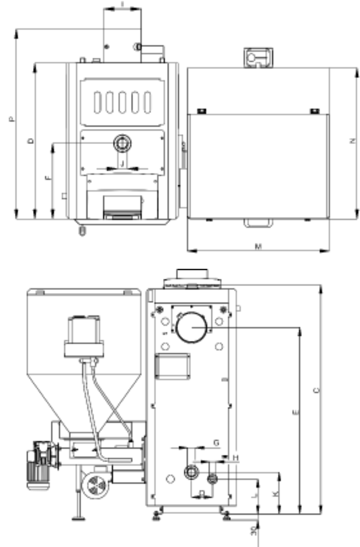
Рисунок 10.1 Размеры котла SEG BIO
