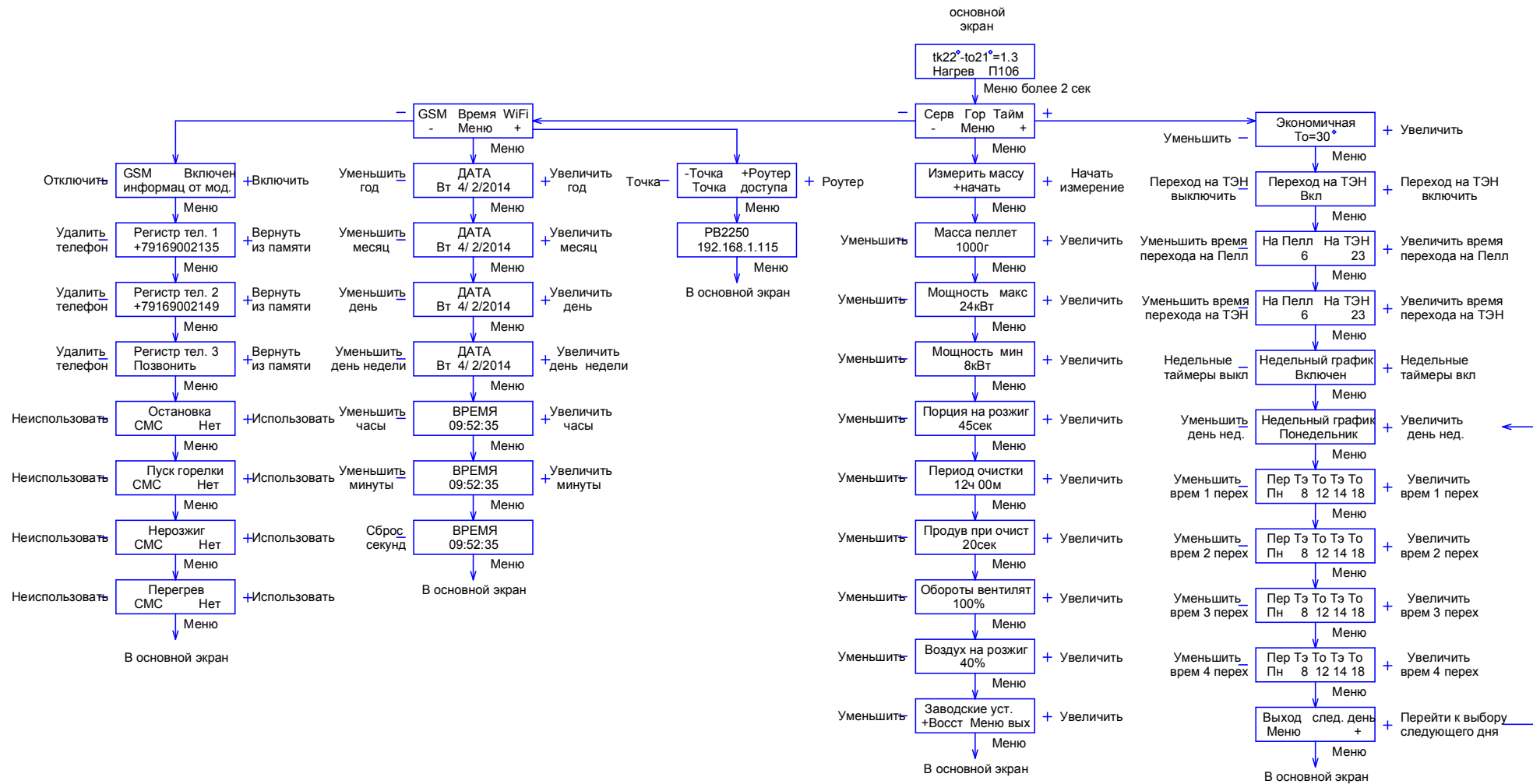
Рис.10. Структура меню наладки.
