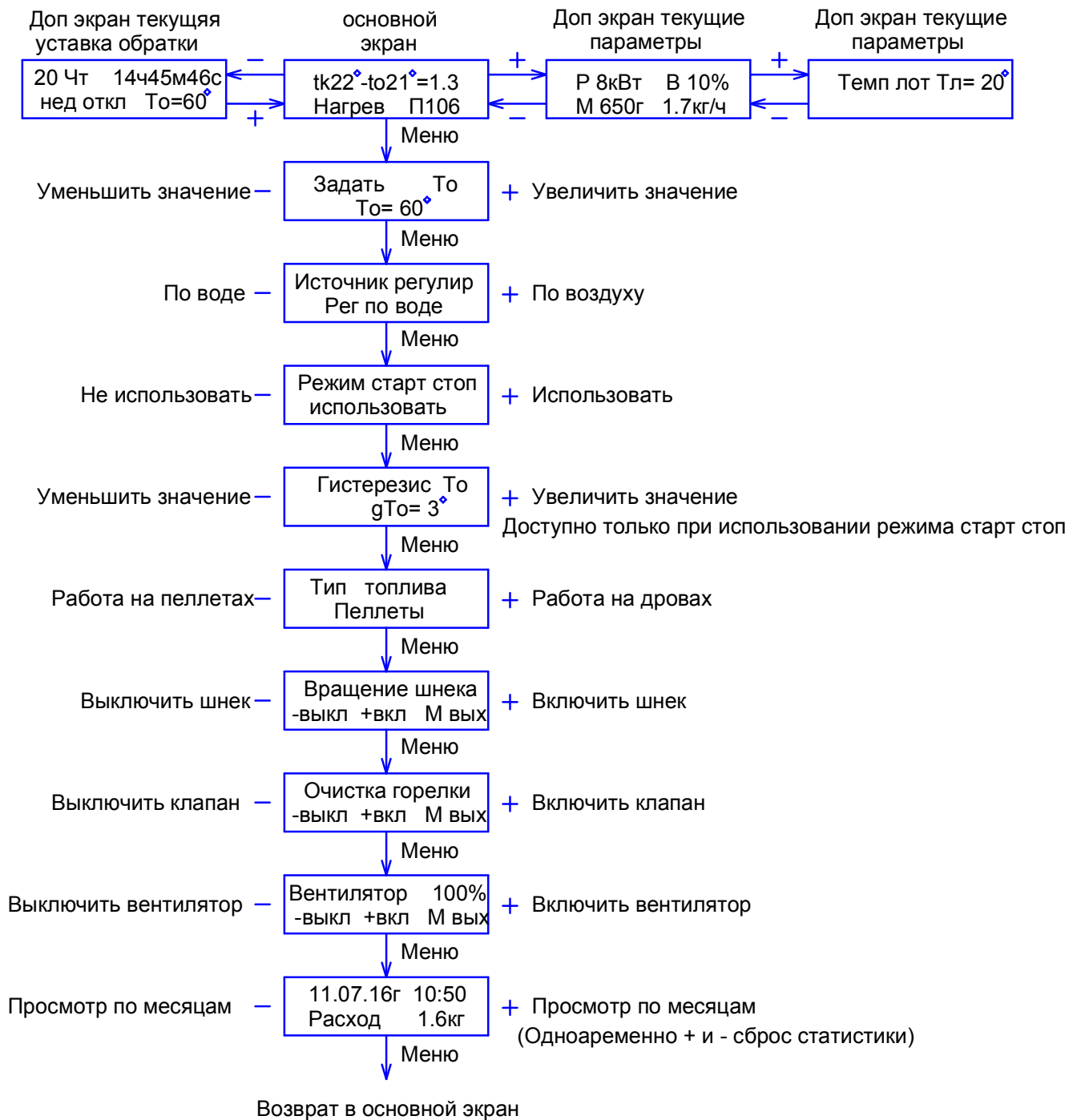
Рис. 9. Меню пользователя.
