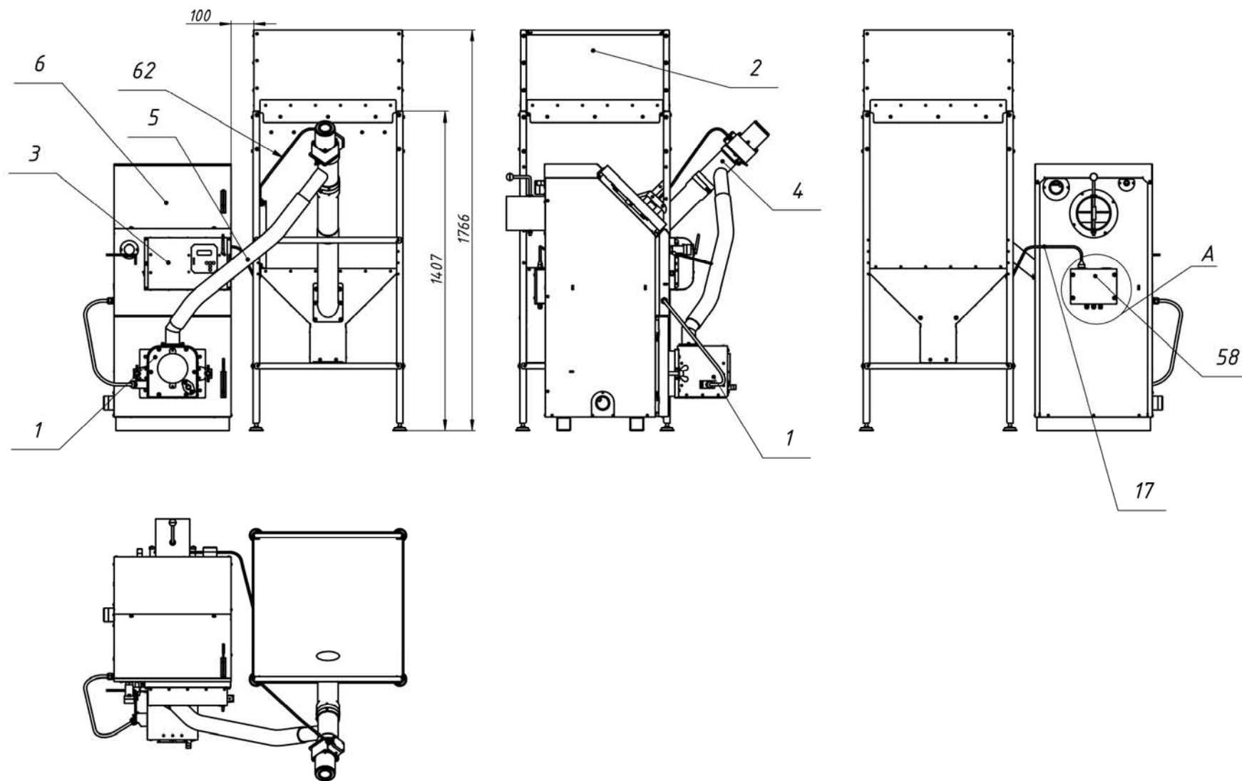
Рис. 1а Размещение горелки на котле.
