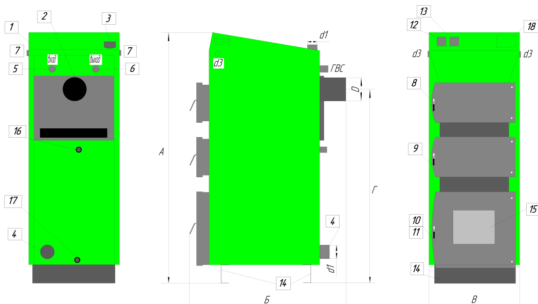
Рисунок 3. Основные размеры котлов Bioten (SBE/SBLE)
